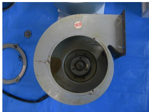
ファンを取り外したモーター部 中央に3つの排熱穴がある
